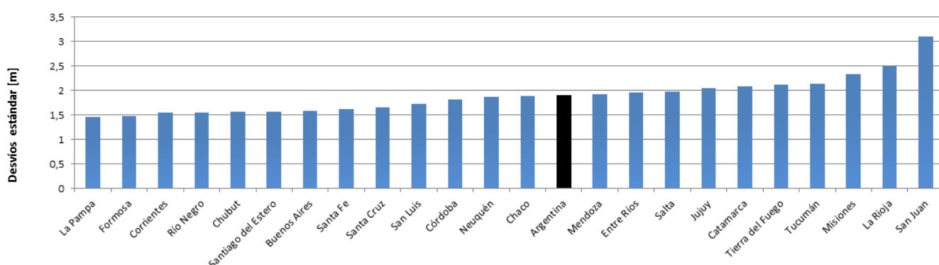
Fig. 17: Desvíos estándar de las diferencias entre las alturas de 24072 puntos altimétricos y las alturas derivadas del MDE-Ar v2.1
