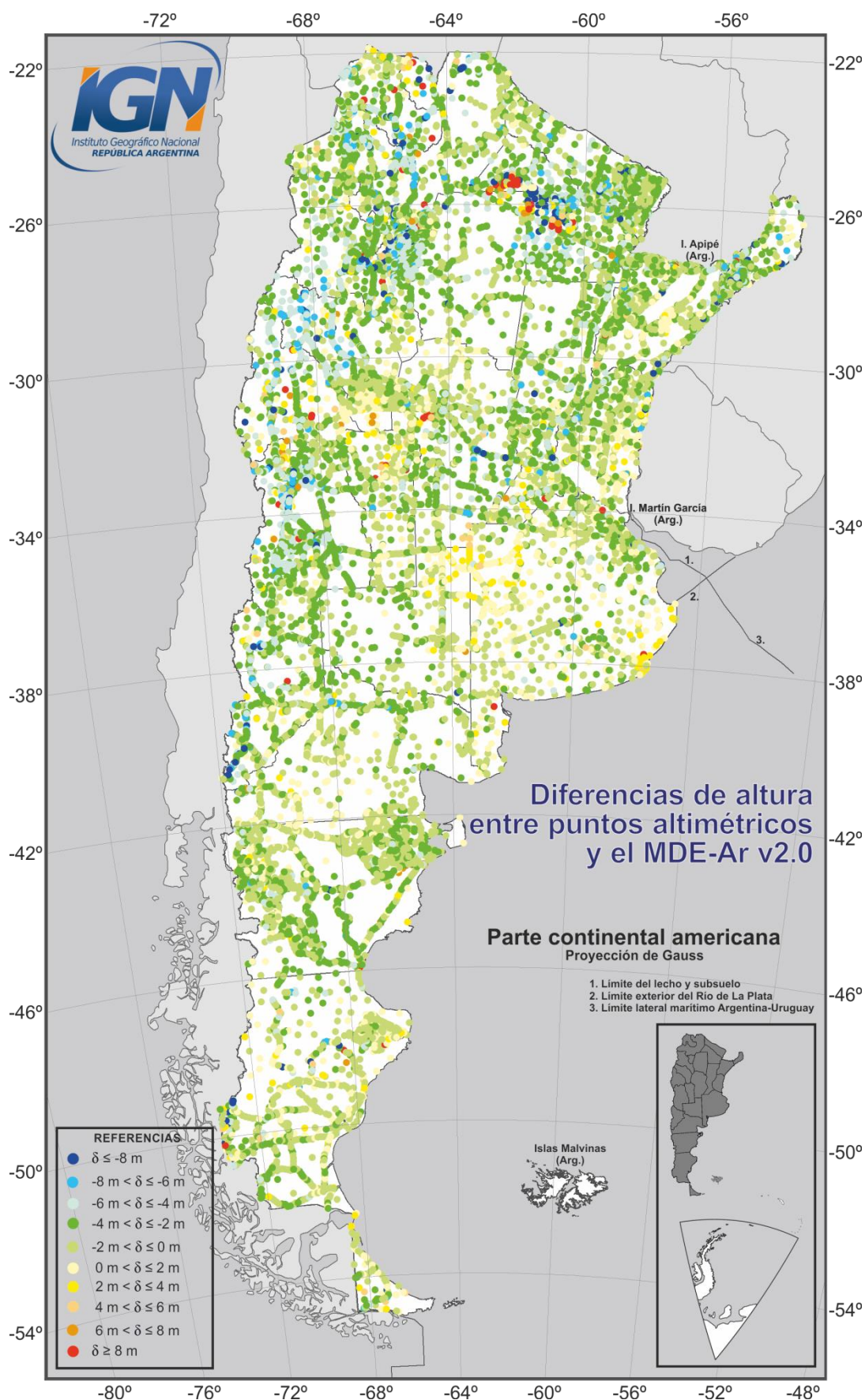
Fig. 10: Diferencias entre las alturas de 23411 puntos altimétricos y las alturas derivadas del MDE-Ar v2.0
