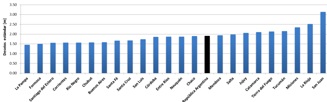
Fig. 9: Desvíos estándar de las diferencias entre las alturas de 23411 puntos altimétricos y las alturas derivadas del MDE-Ar v2.0
