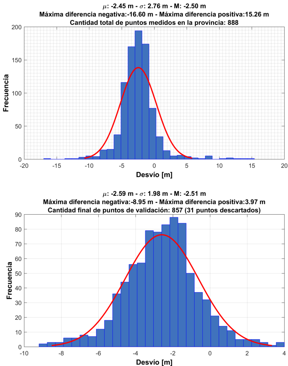
Fig. 35: Histograma de las diferencias entre las alturas de los puntos alimétricos y las alturas derivadas del MDE-Ar v2.1 en la Provincia de Salta
