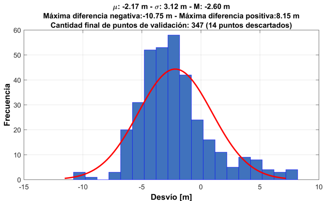
Fig. 36: Histograma de las diferencias entre las alturas de los puntos altimétricos y las alturas derivadas del MDE-Ar v2.1 en la Provincia de San Juan
