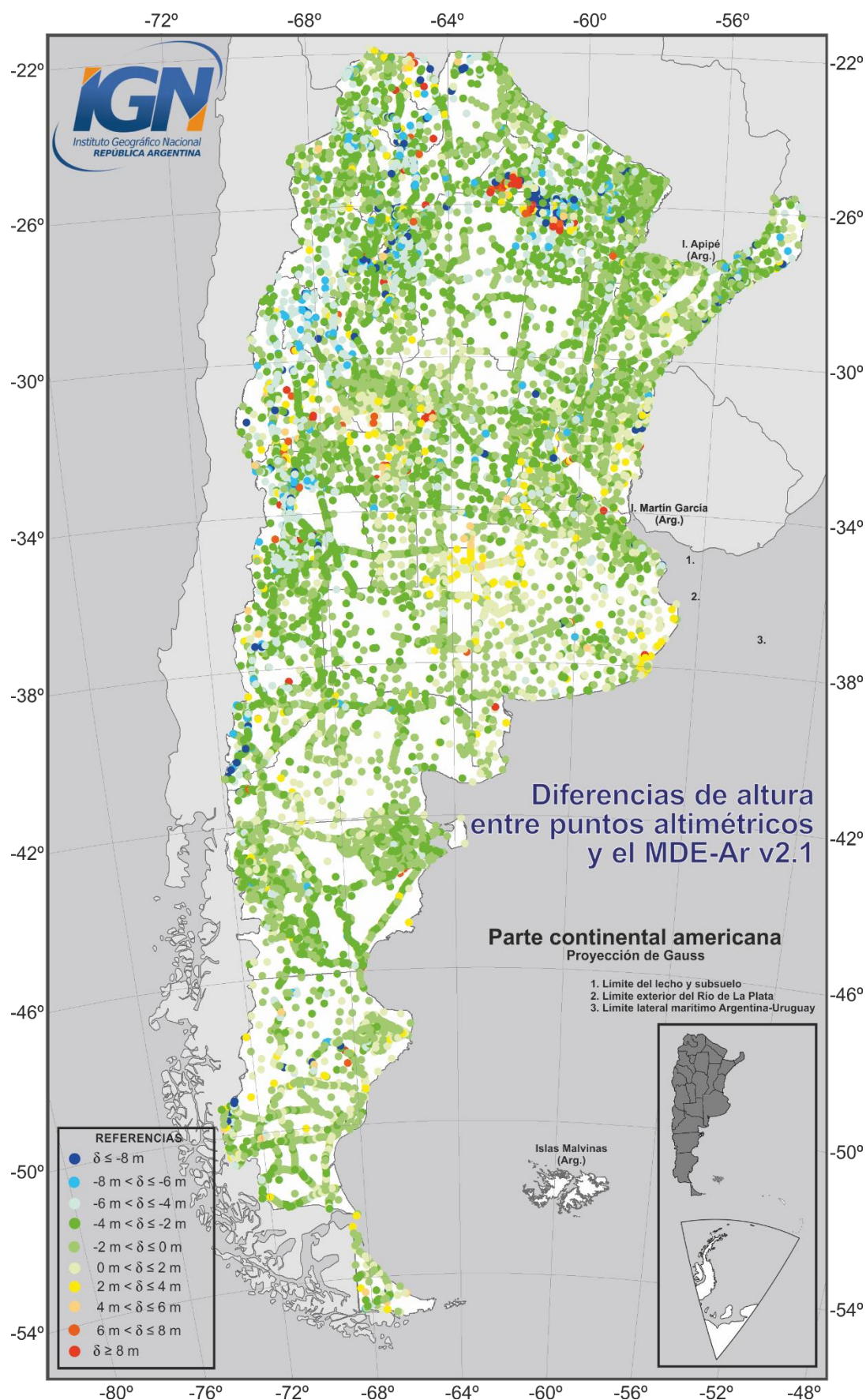
Fig. 18: Diferencias entre las alturas de 24072 puntos altimétricos y las alturas derivadas del MDE-Ar v2.1
