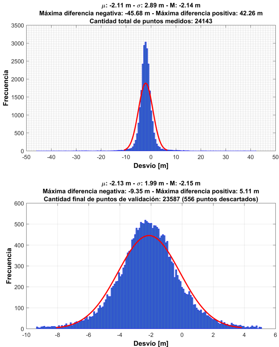
Fig. 11: Histograma de las diferencias entre las alturas de los puntos altimétricos y las alturas derivadas del MDE-Ar v2.0 en la República Argentina
