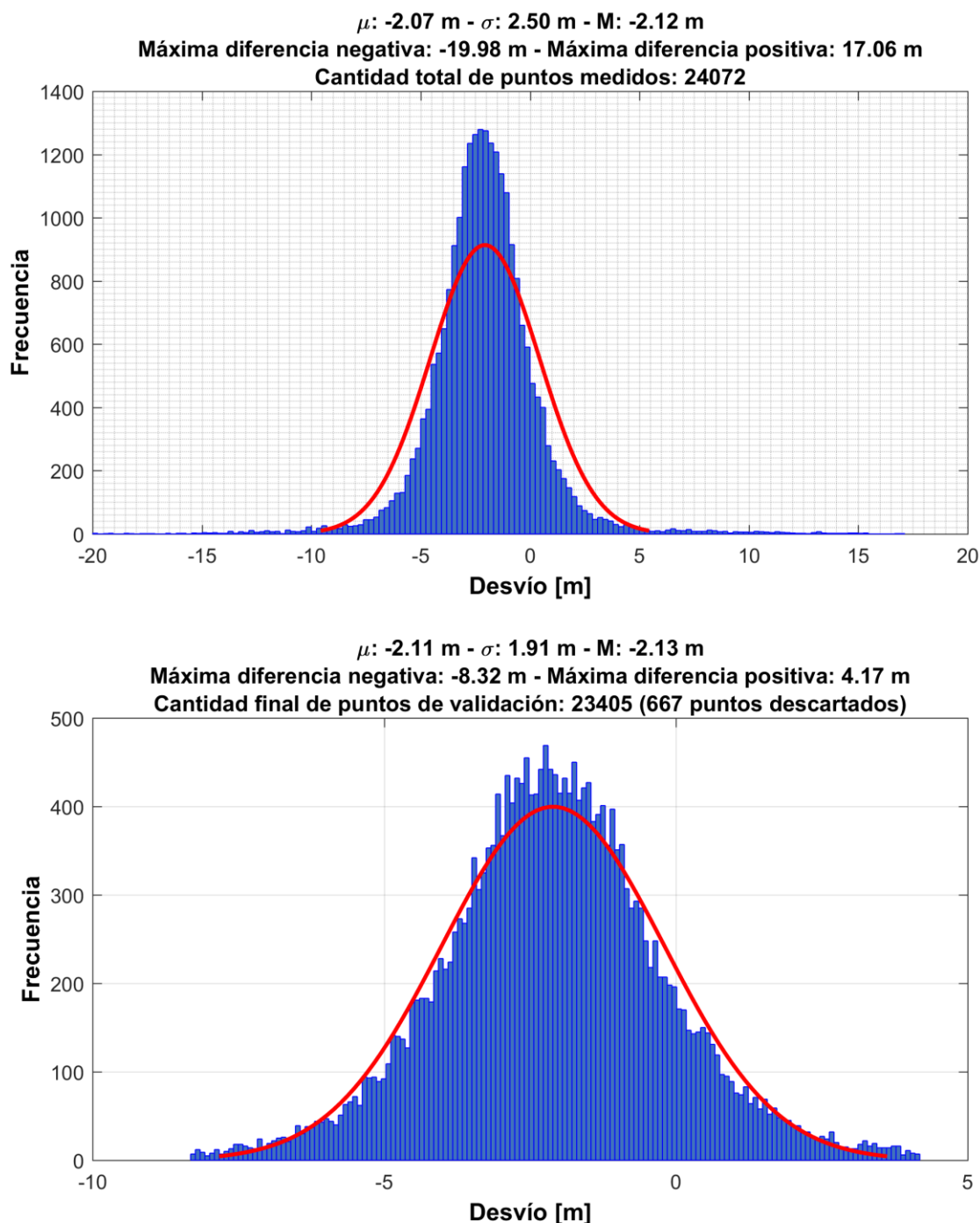
Fig. 19: Histograma de las diferencias entre las alturas de los puntos altimétricos y las alturas derivadas del MDE-Ar v2.1 en la República Argentina
